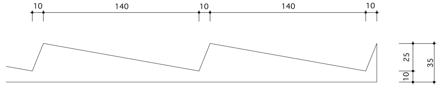
拡大断面図
