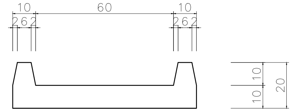
b-b断面図
