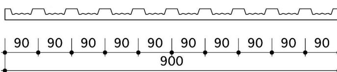
(製品図)
