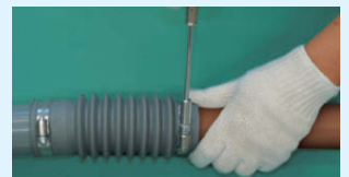
銅管接続 (バンド締め) 完成
