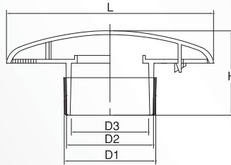
ソケット付 \phi 65VU用 (ABS樹脂製)
