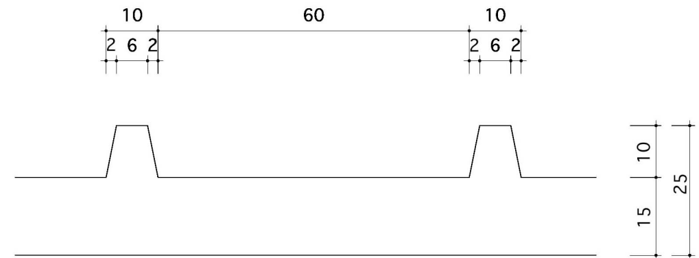
b-b断面図
