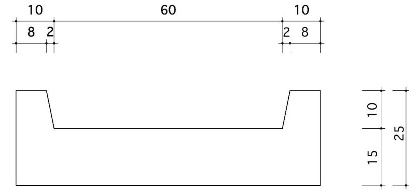
a-a断面図
