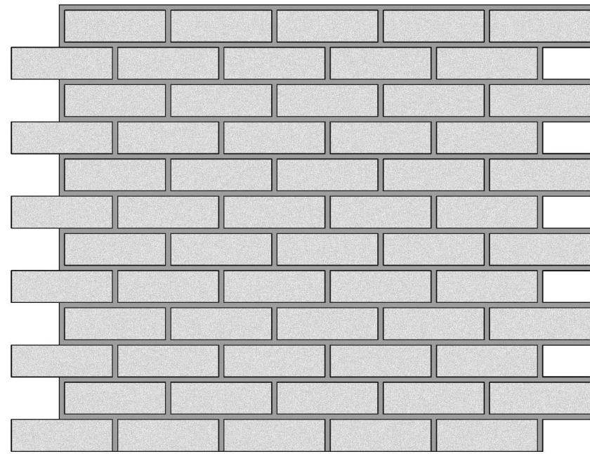
(仕上図)
