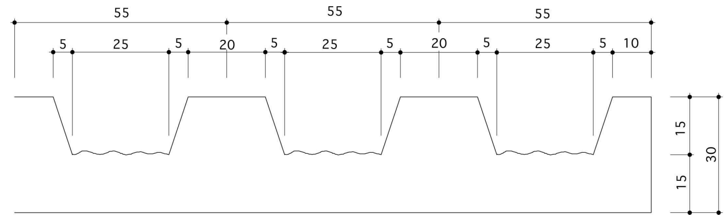
横拡大断面図 S=1/1
