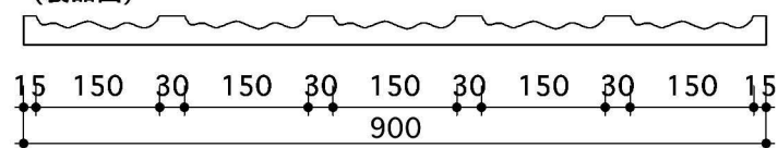
(製品図)
