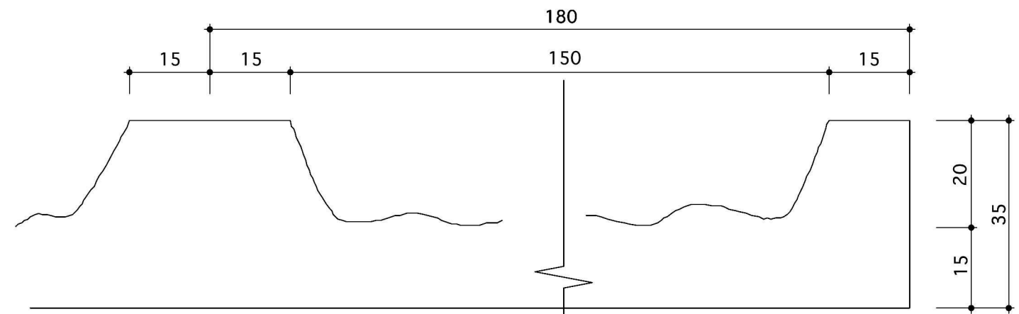
横拡大断面図 S=1/1
