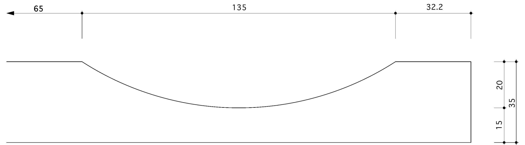
拡大断面図 S=1/1
