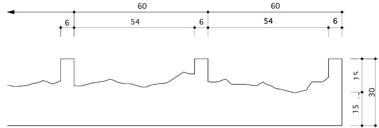
b-b断面
