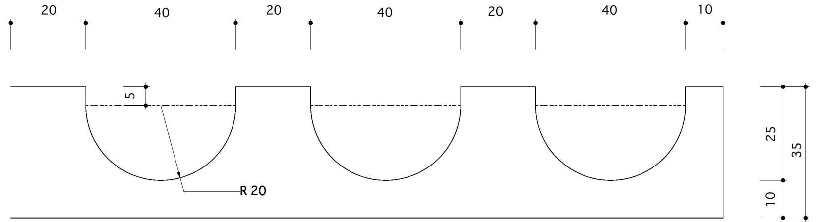
拡大断面図
