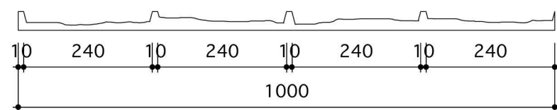
(製品図)
