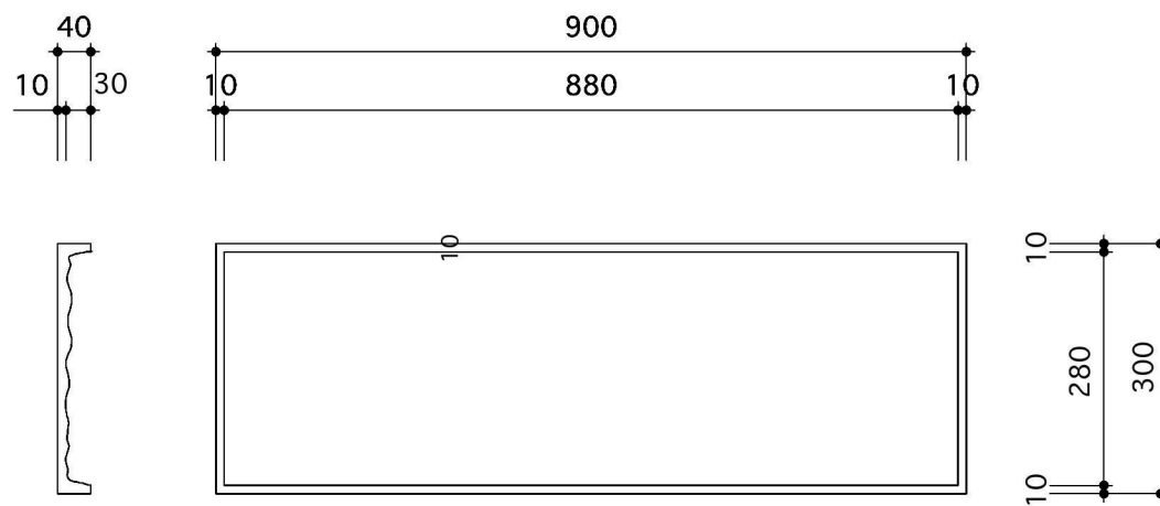
(製品図)
