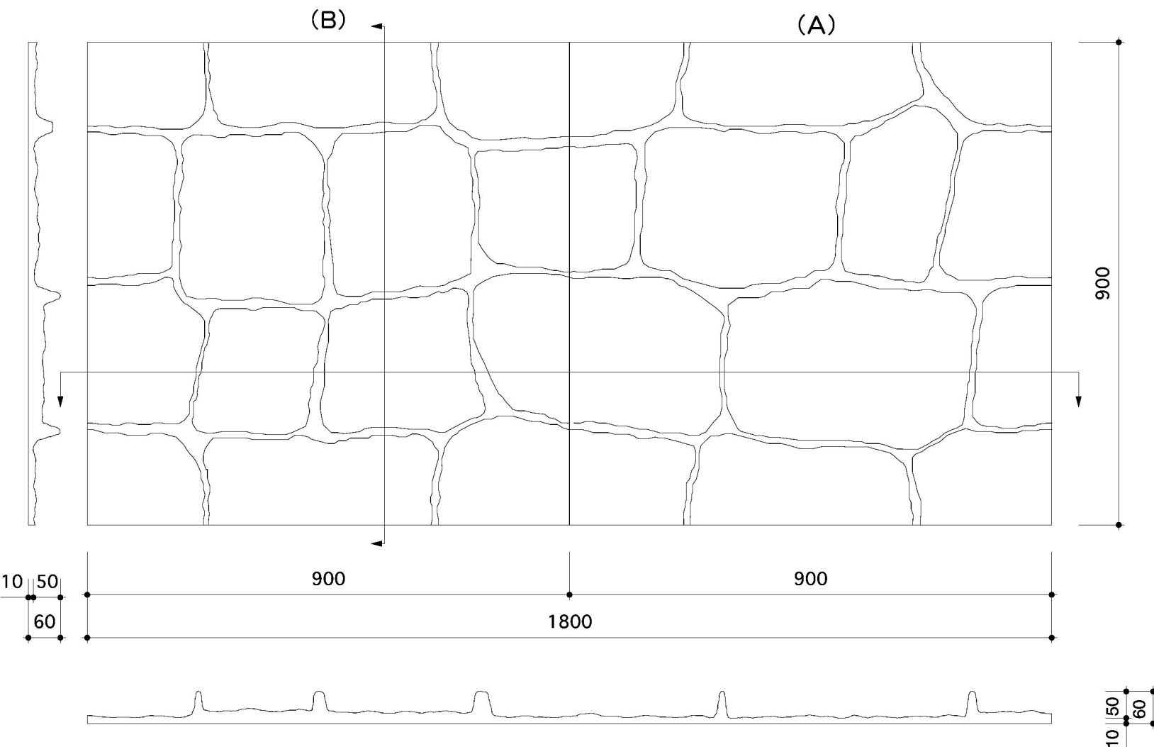
2)細い目地詳細
