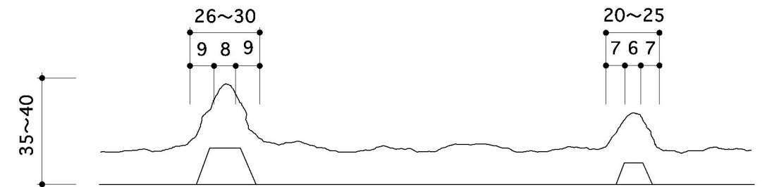
拡大断面図 S=1/2
