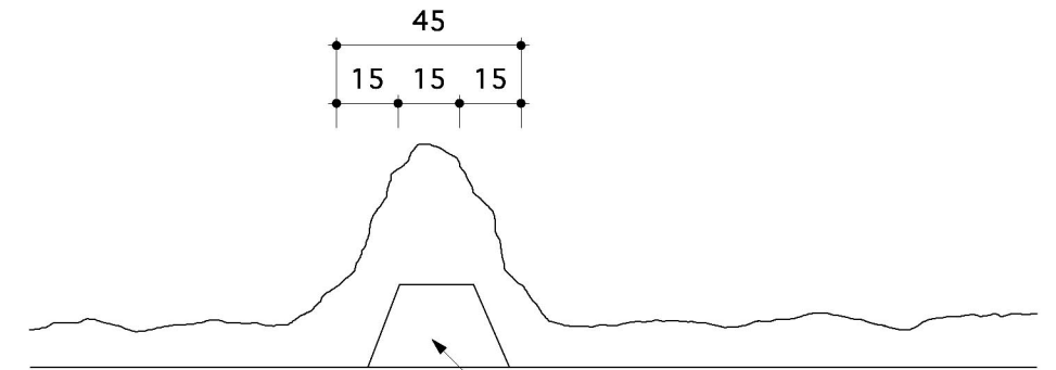
1)太い目地詳細
