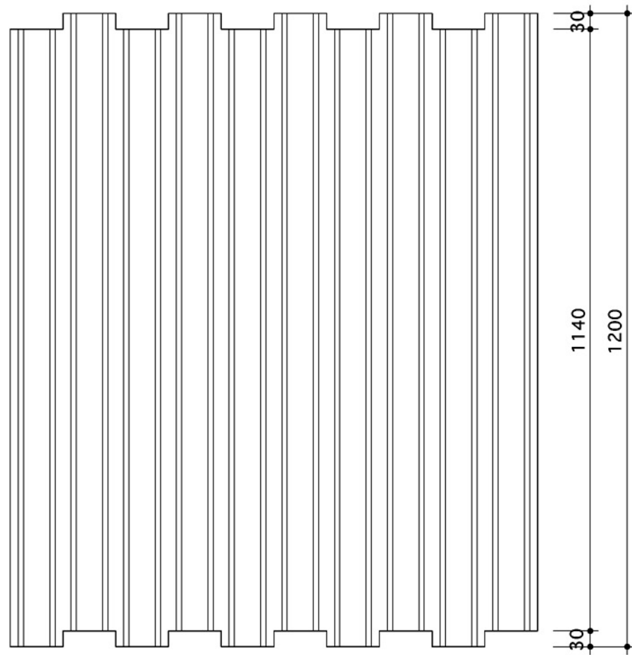
(製品図)
